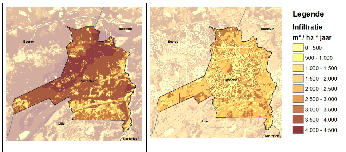
Figuur 12: Potentiële infiltratie (links) t.o.v. de actuele infiltratie (rechts) xxiii
