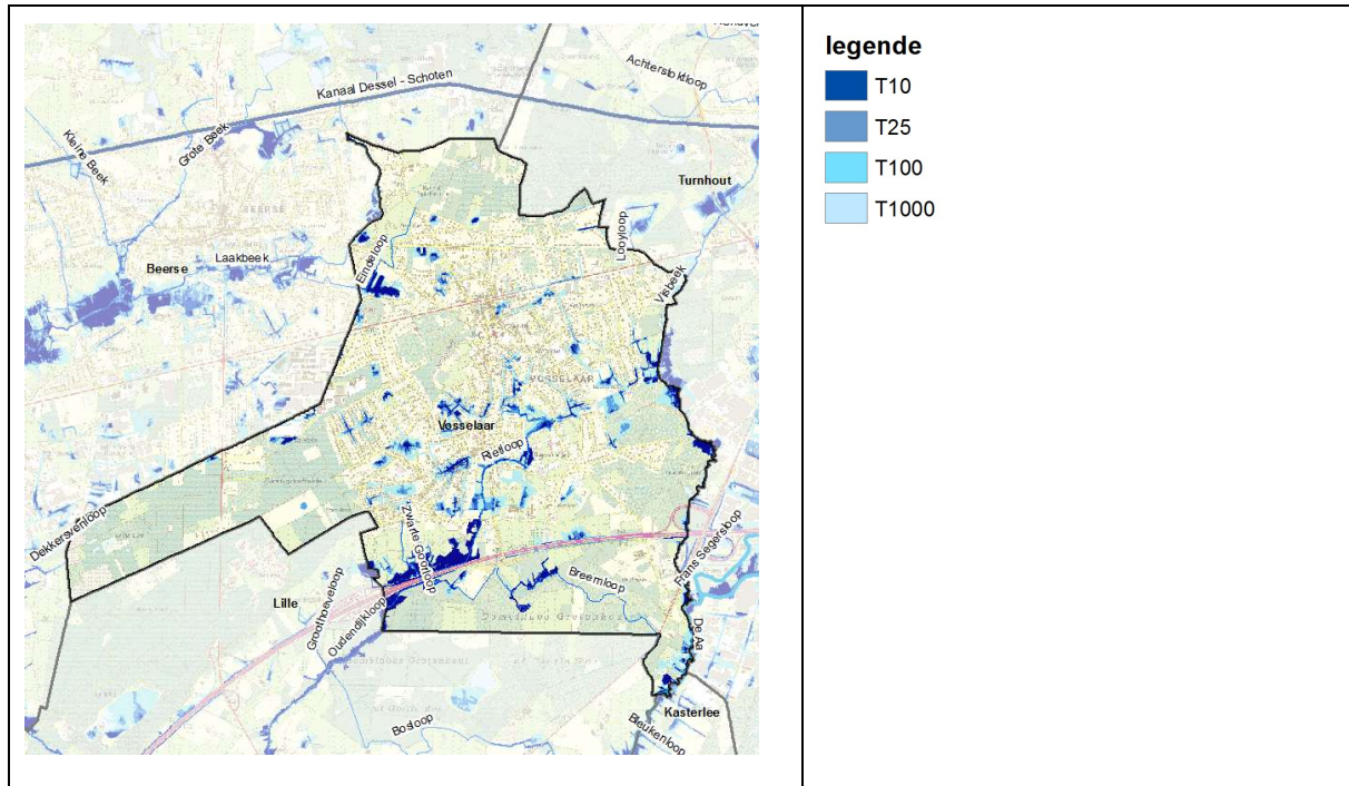
Figuur 16: Pluviale overstromingskaart Vosselaar xxx
