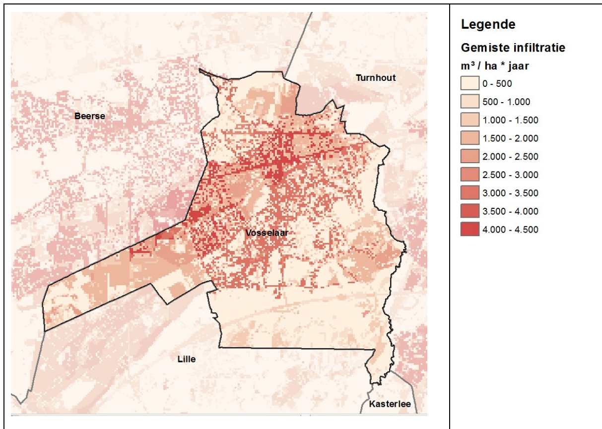
Figuur 13: Niet-gerealiseerde infiltratie xxiv
