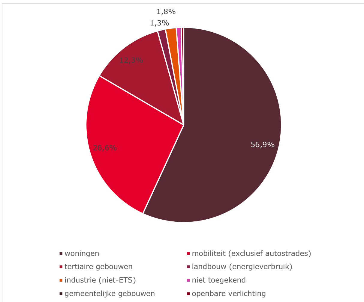
Figuur 1: Bronnen van CO 2 -uitstoot in Vosselaar in 2018
