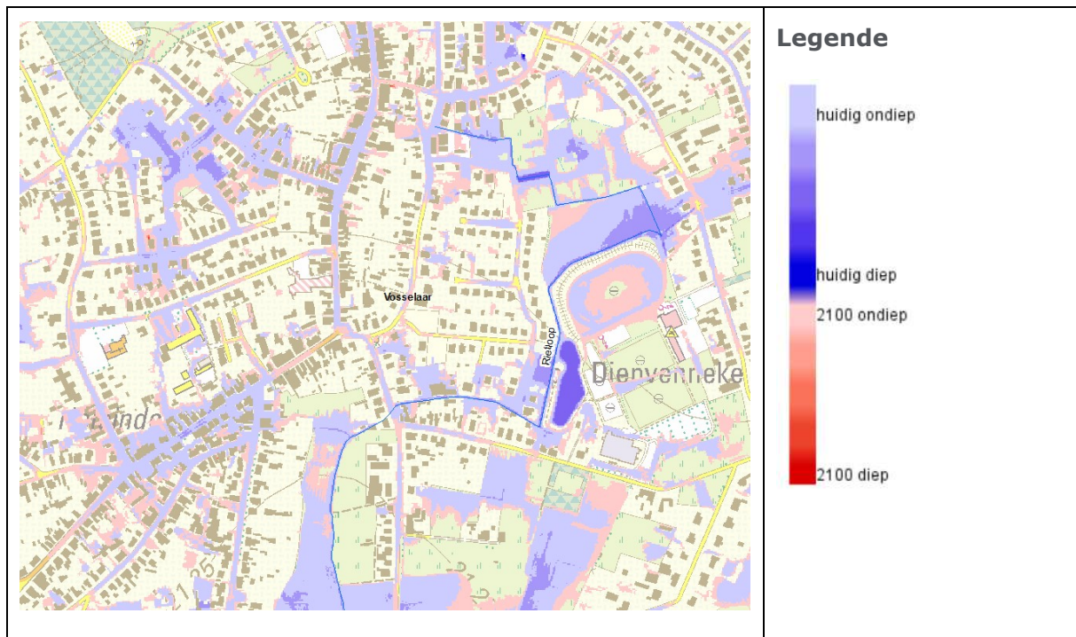
Figuur 15 : Aangroei overstroombaar gebied in de omgeving van Vosselaar xxviii
