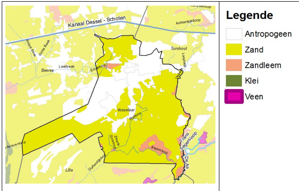
Figuur 5: Vereenvoudigde bodemkaart
