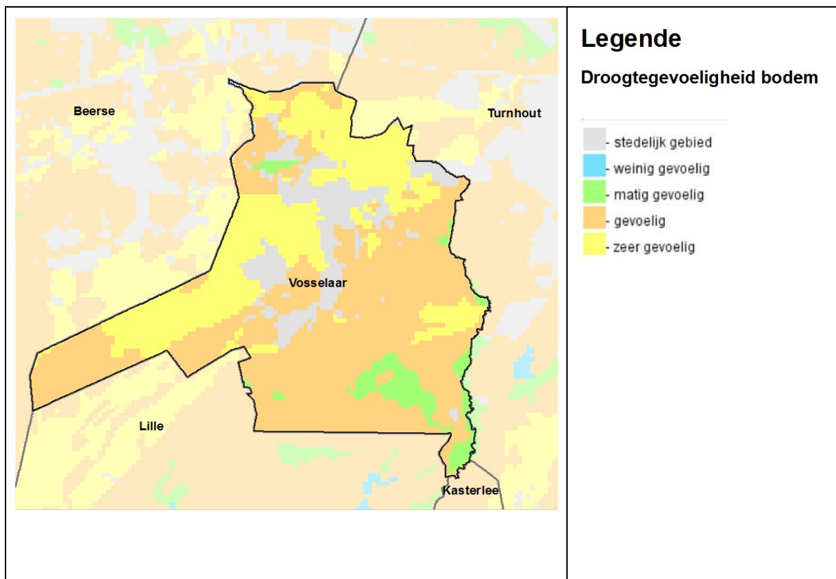
Figuur 10: Droogtegevoeligheid bodem xxi
