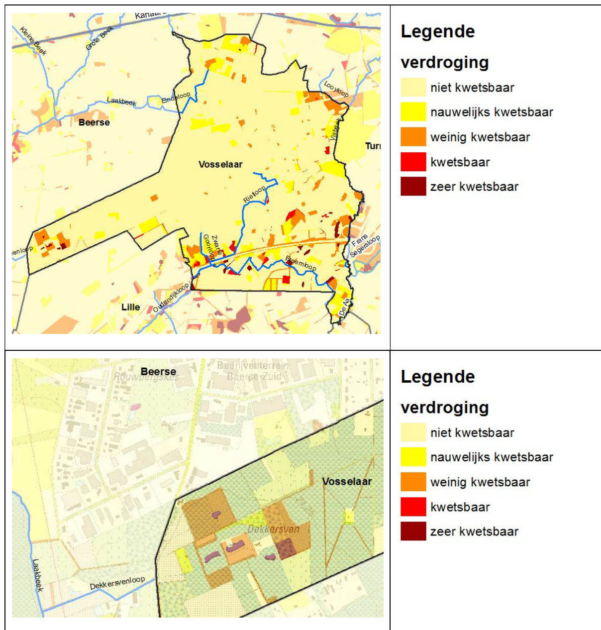
Figuur 11 : Ecotoopkwetsbaarheidskaart van de gemeente met detail
