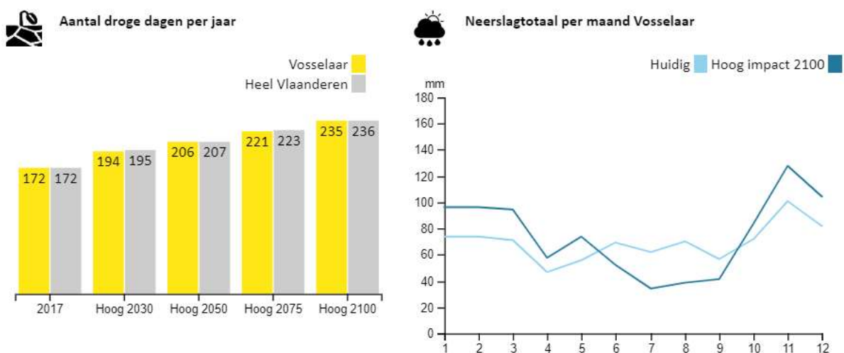
Figuur 9 Evolutie van het aantal droge dagen en spreiding van neerslag xix
