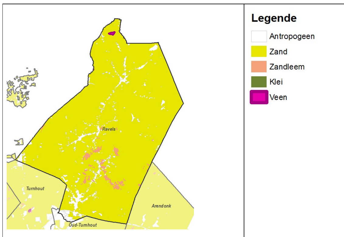
Figuur 5: Vereenvoudigde bodemkaart
