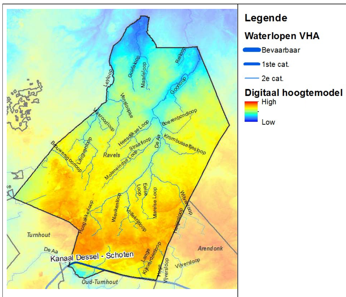
Figuur 4: Digitaal hoogtemodel met geklasseerde waterlopen
