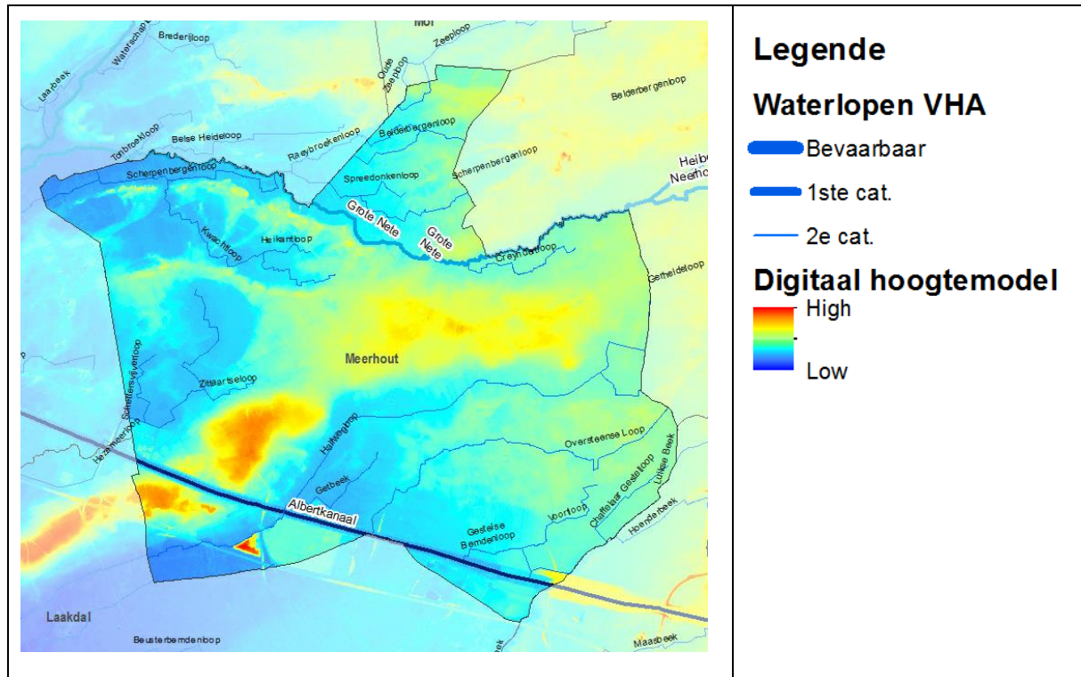
Figuur 4: Digitaal hoogtemodel met geklasseerde waterlopen
