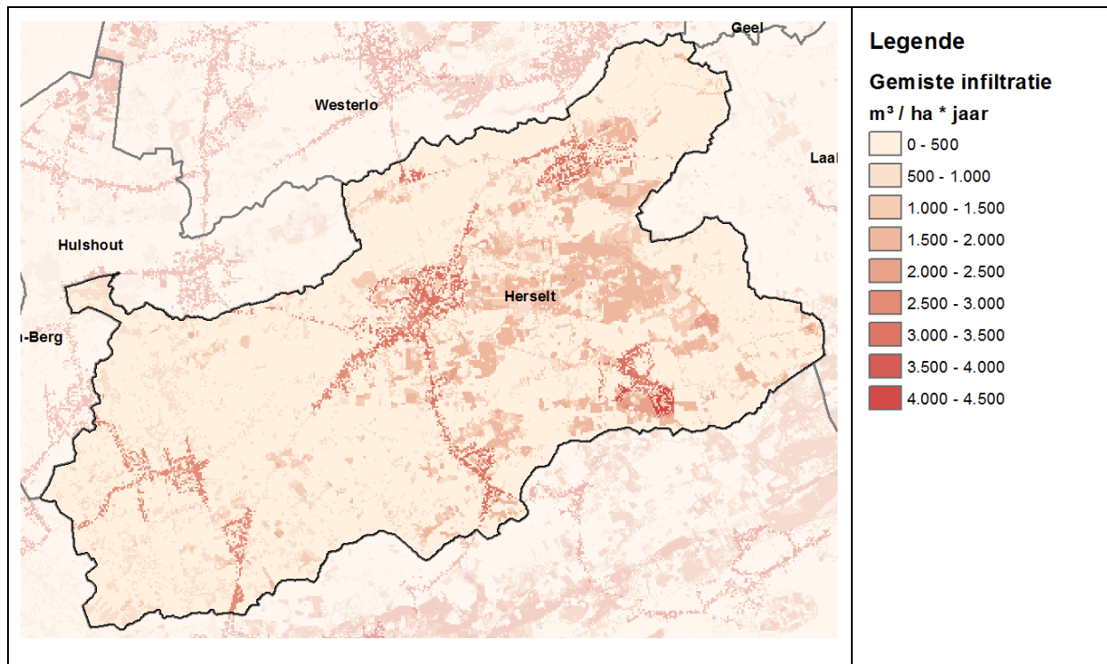
Figuur 12: Niet-gerealiseerde infiltratie xxv
