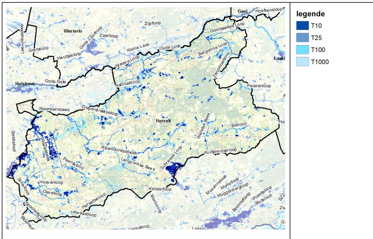
Figuur 15: Pluviale overstromingskaart Herselt xxx
