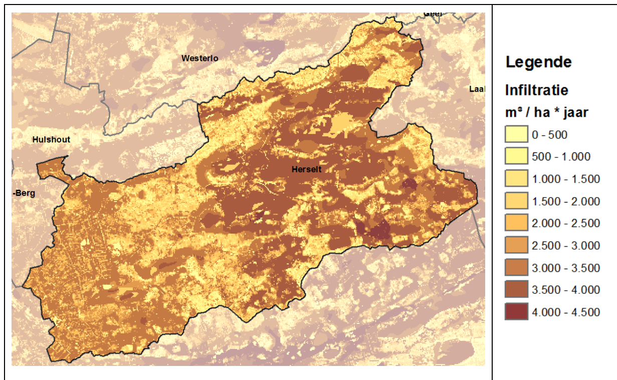
Figuur 11: Potentiële infiltratie (boven) t.o.v. de actuele infiltratie (onder) xxiv
