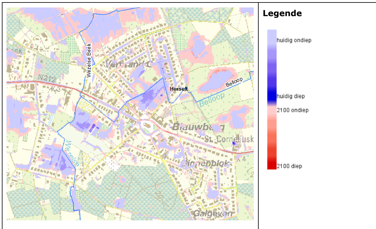
Figuur 14 : Aangroei overstroombaar gebied ter hoogte van Blauwberg xxviii
