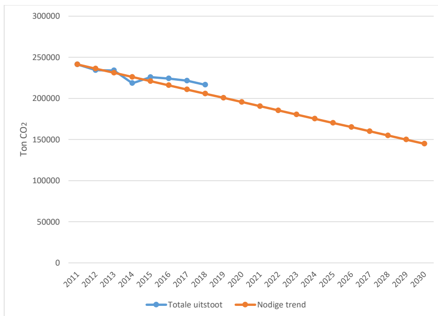
Figuur 2: Evolutie CO 2 -uitstoot Geel en nodige trend om klimaatdoel te halen
