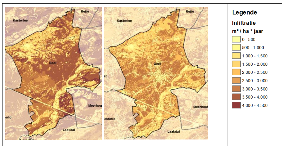
Figuur 14: Potentiële infiltratie (links) t.o.v. de actuele infiltratie (rechts) xxiii
