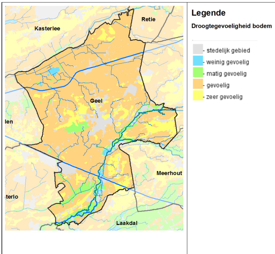
Figuur 12: Droogtegevoeligheid bodem xxi
