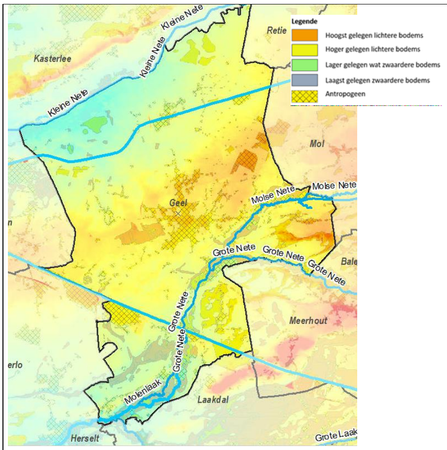
Figuur 7 : Samenvattende kaart
