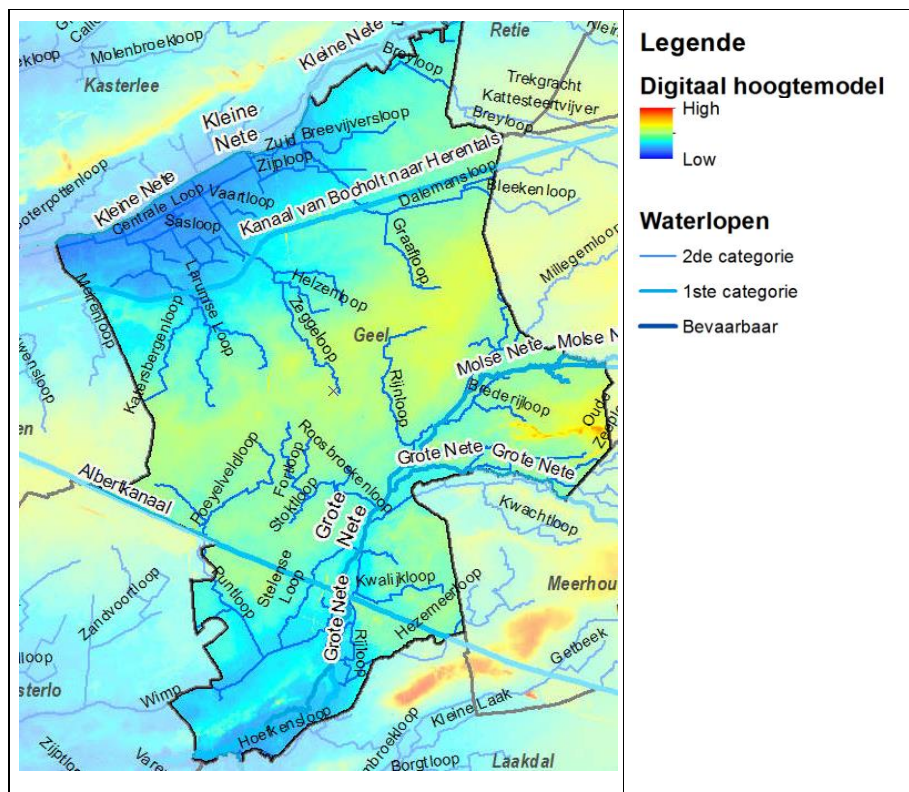
Figuur 5: Digitaal hoogtemodel met geklasseerde waterlopen
