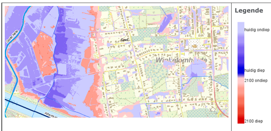
Figuur 17 : Aangroei overstroombaar gebied in de vallei van de Grote Nete thv Winkelomheide (voorbeeld) xxvii
