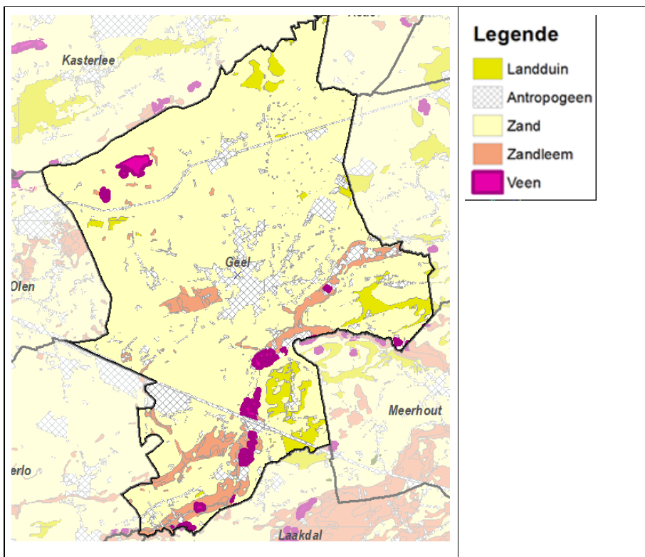
Figuur 6: Vereenvoudigde bodemkaart
