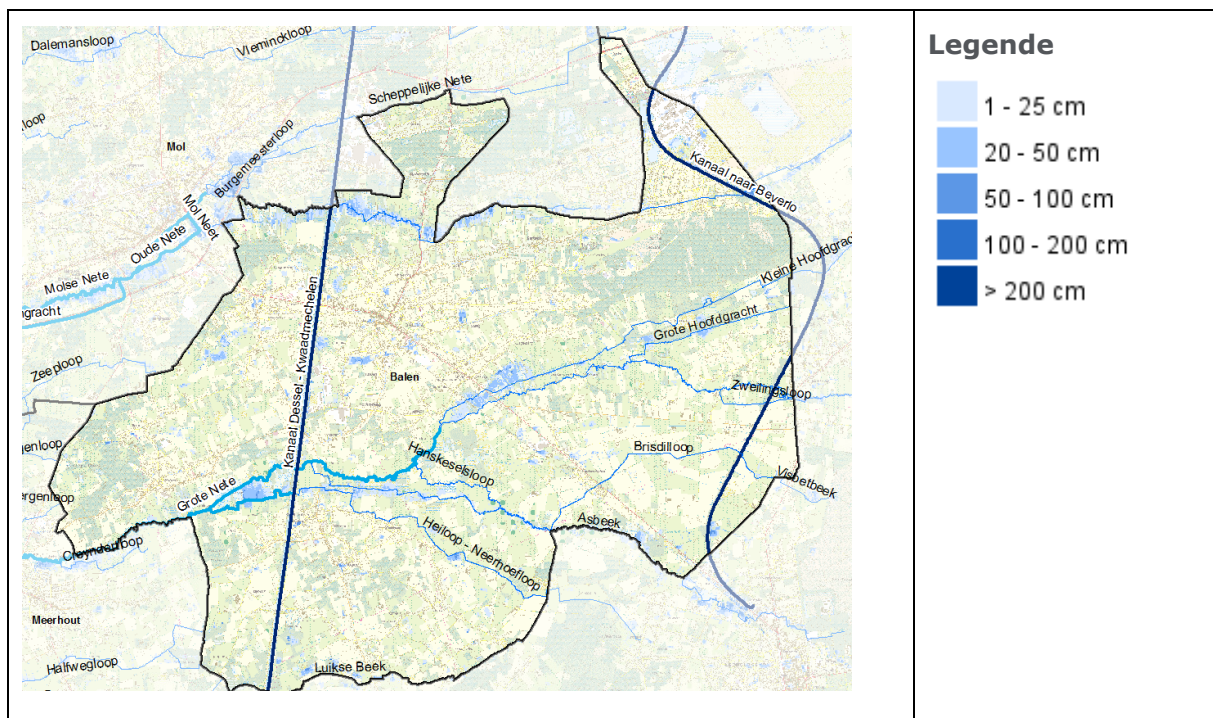
Figuur 16: Overstromingsgevaarkaart : waterdiepte riooloverstroming bij T100 xxxi
