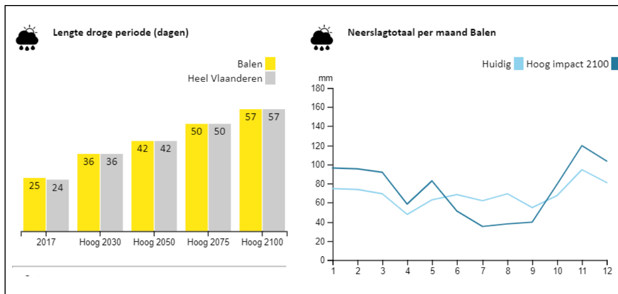
Figuur 10 Evolutie van de lengte van droge periode en spreiding van neerslag xx
