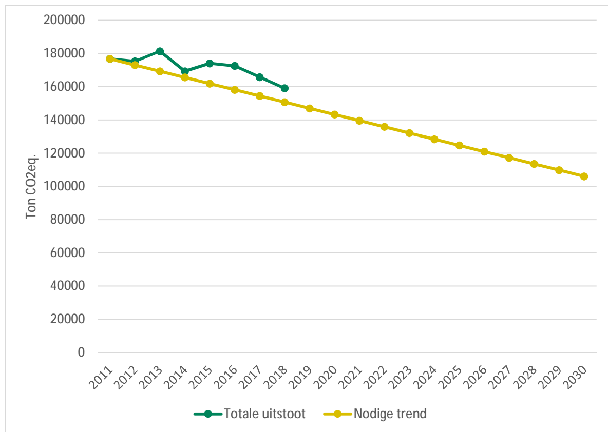
Figuur 2: Evolutie CO 2 -uitstoot Mol en nodige trend om klimaatdoel te halen
