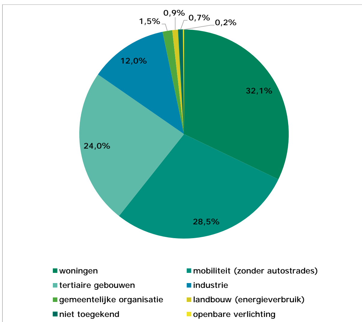
Figuur 1: Bronnen van CO 2 -uitstoot in Mol in 2018
