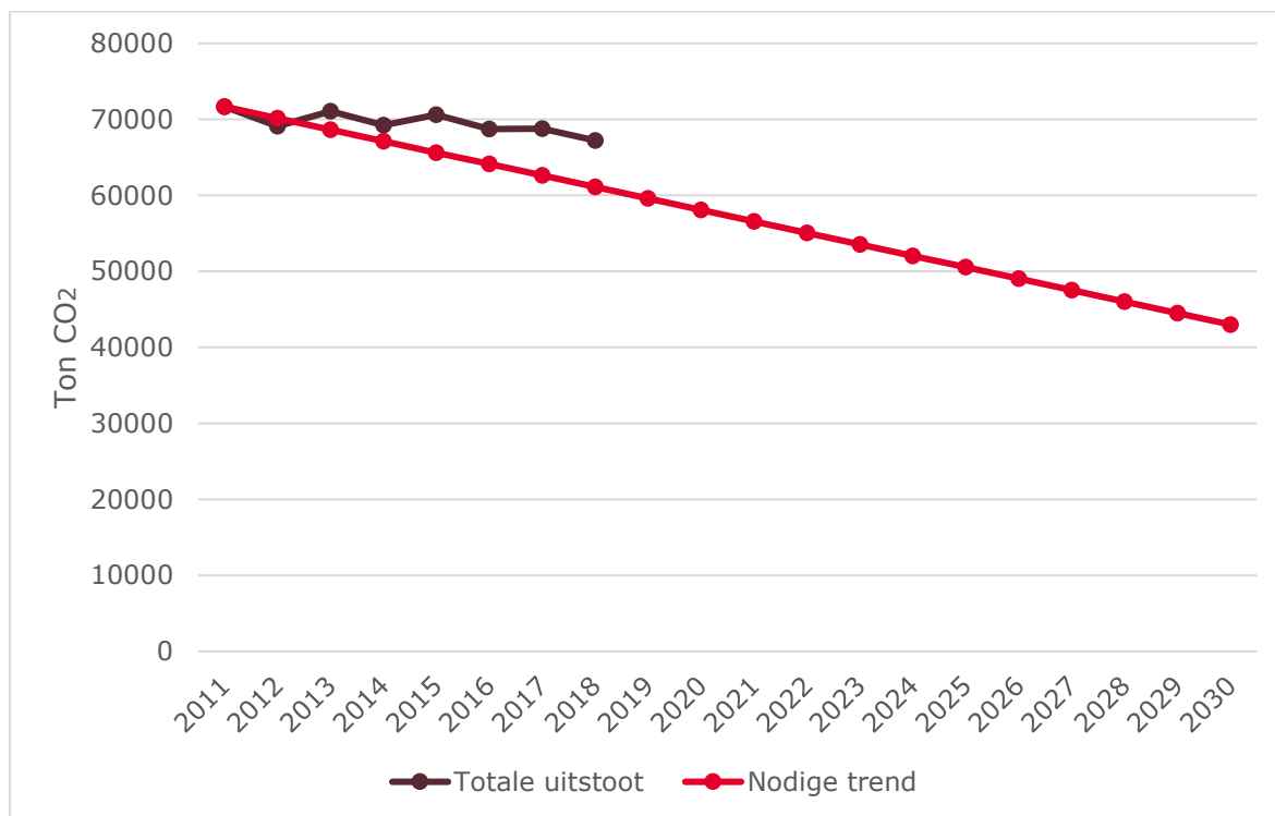
Figuur 2: Evolutie CO 2 -uitstoot Nijlen en nodige trend om klimaatdoel te halen
